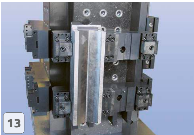
84 Teile sind gespannt mit Micro Clamp und werden jeweils nachts unbemannt produziert 84 parts are clamped with Micro Clamp and are machined always at night unmanned
